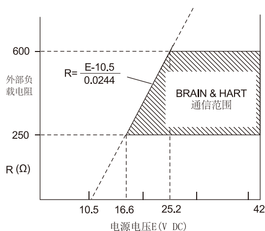
图1. 电源电压与外部负载关系图
